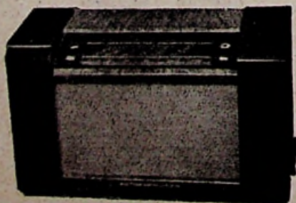
Aetherkruiser superheterodyne A K 1473 van de Algemeene Nederlandsche Radio Unie te Amsterdam.
