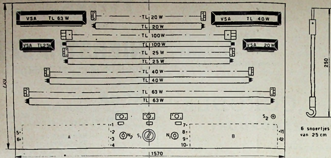
Afb. 1. Schematische voorstelling van het testpaneel.
