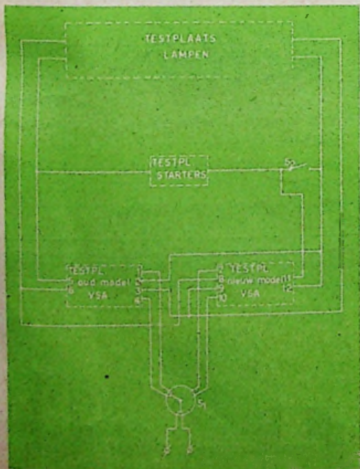
Afb. 2. Principeschema van het testpaneel.
